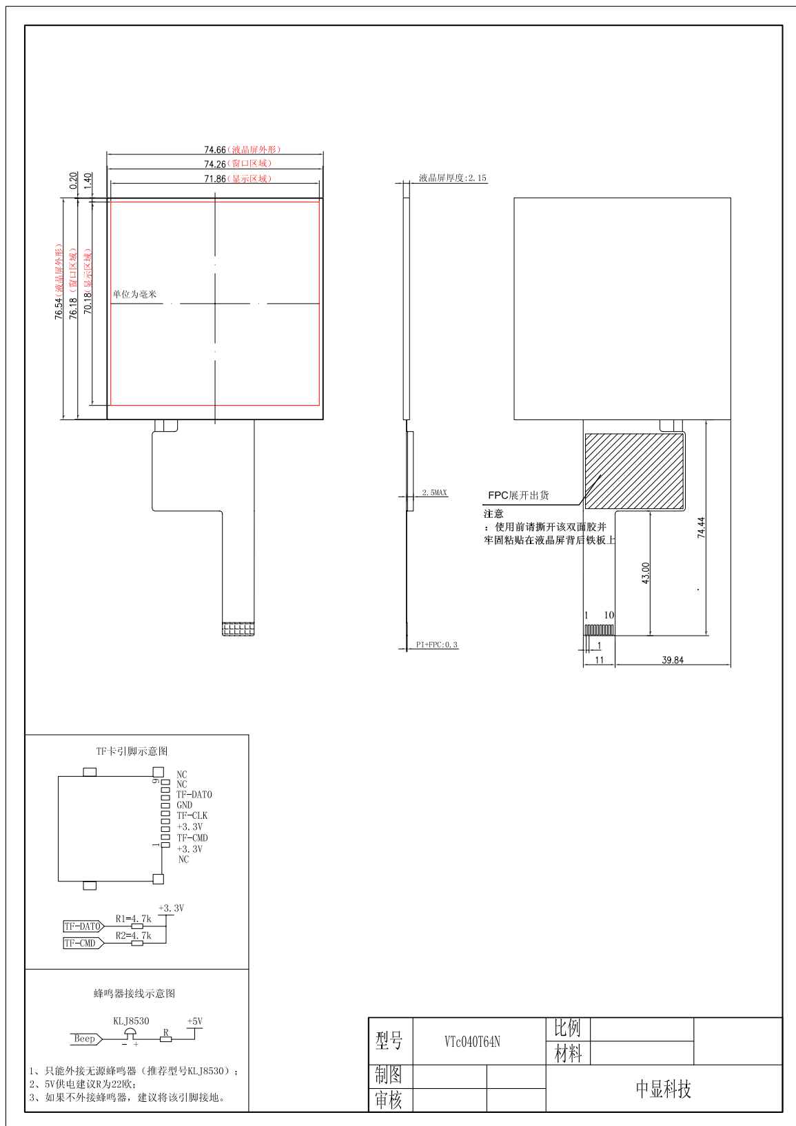
图 2 VTc040T64N 尺寸图
