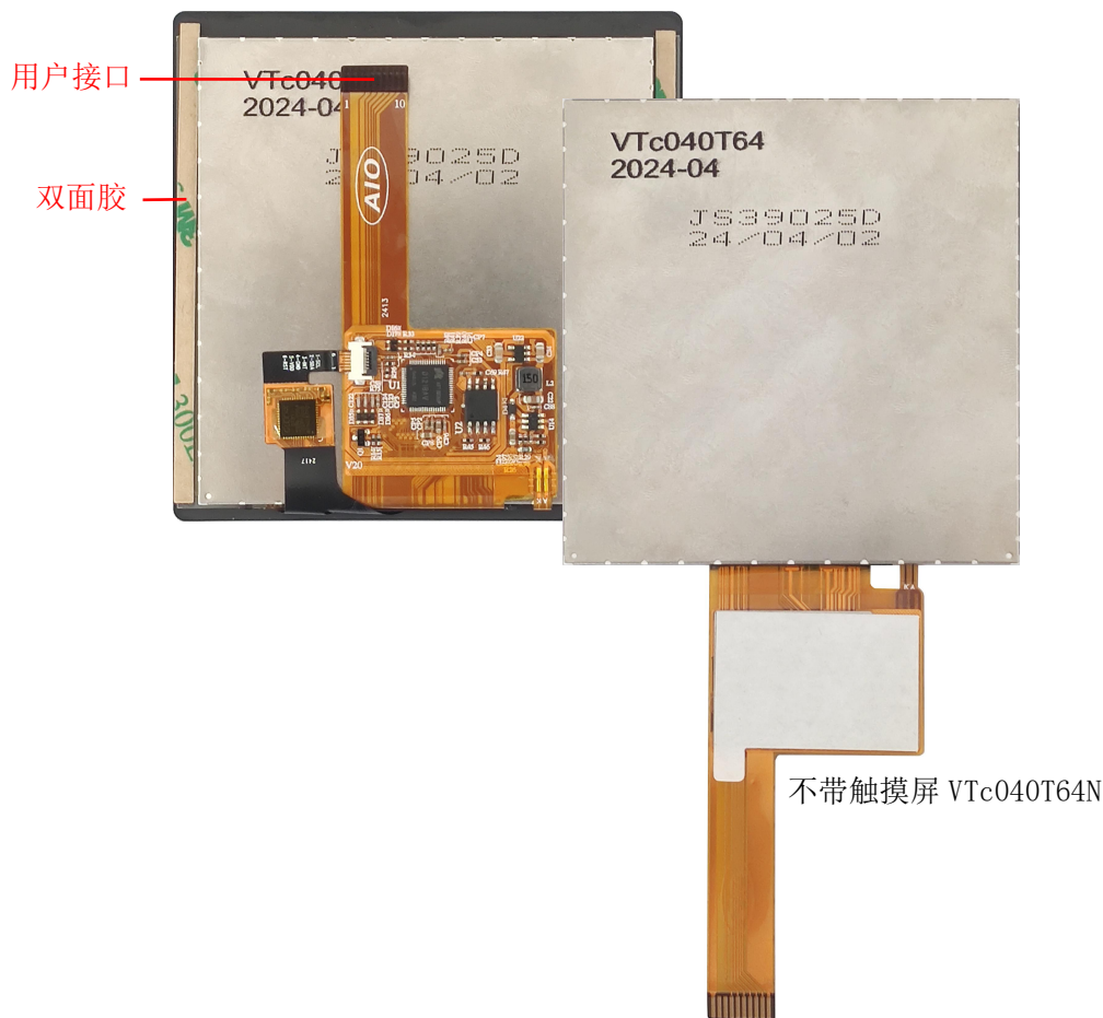
图 1 产品外观及硬件配置图
